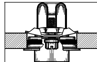
Figure 3 - Chauffe-bloc bien serré dans le bloc.
