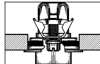
Figure 2 - Chauffe-bloc fermement placé contre le bloc.
